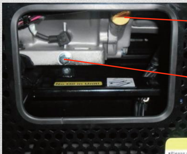
空壓機機油排放口
